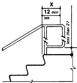
(d) Extension at Top of Run
