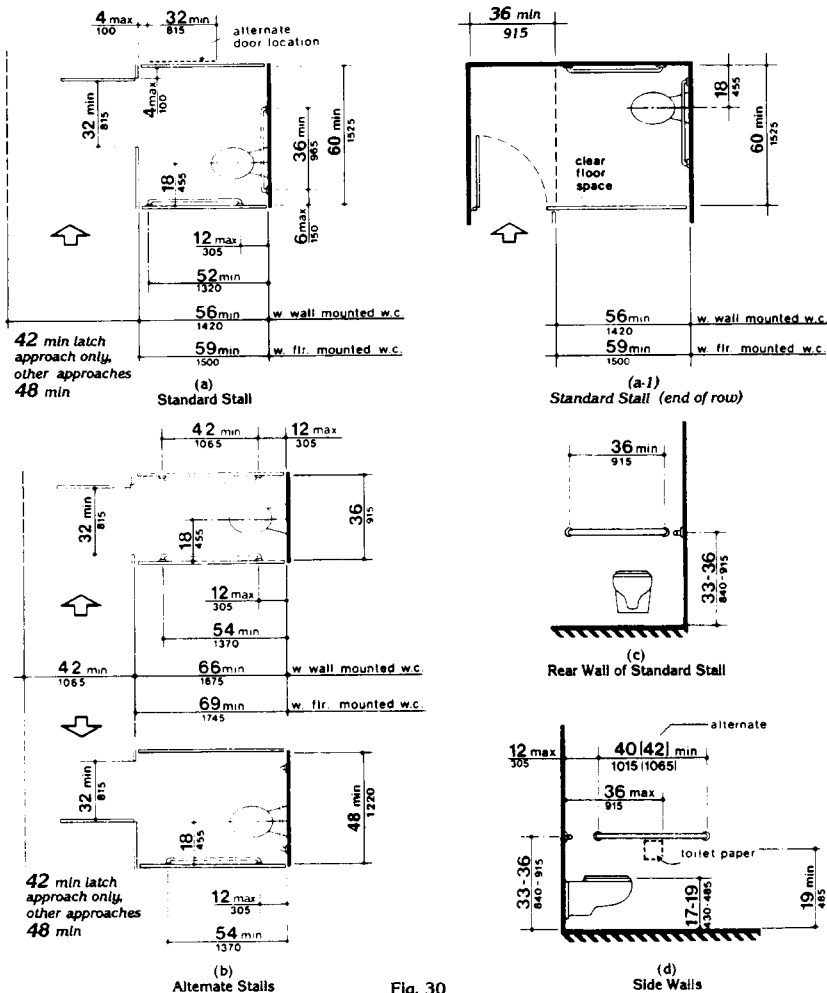
Fig. 30 Toilet Stalls
