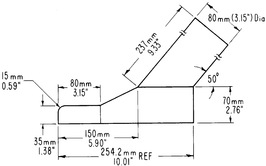
FIG 2—FOOT PROBE
