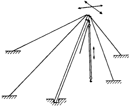
GIN POLE
